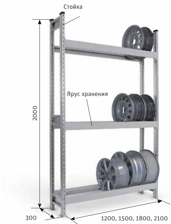
Стеллаж СТ-023 для автомобильных дисков
