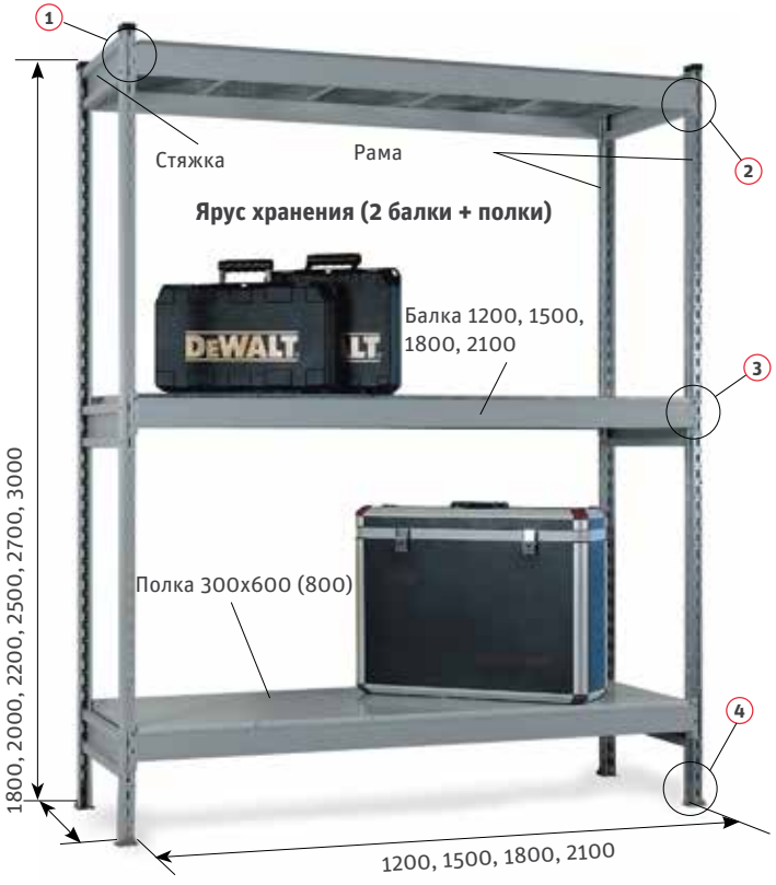
Стеллаж СТ-023
