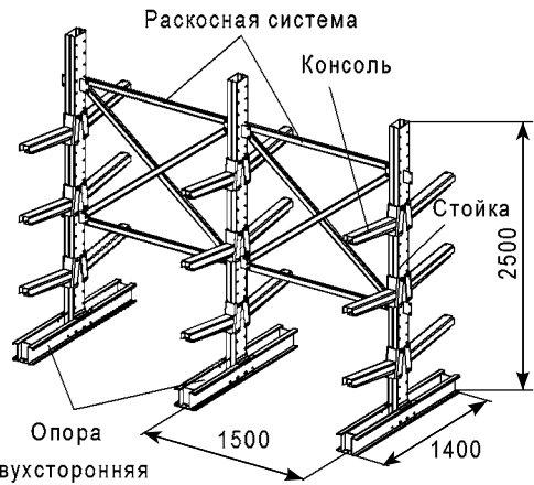
СТ-062 Стеллаж двухсторонний
