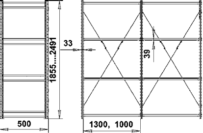
Схема вариантов установки стеллажей СТ-031
