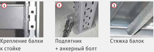
Элементы стеллажа СТ-051
