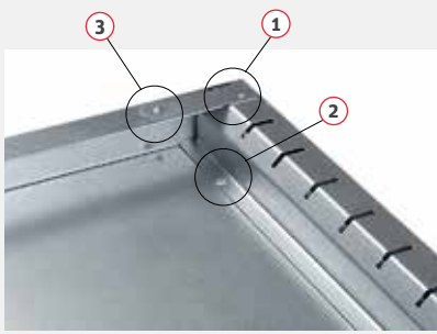
Вид полки изнутри
